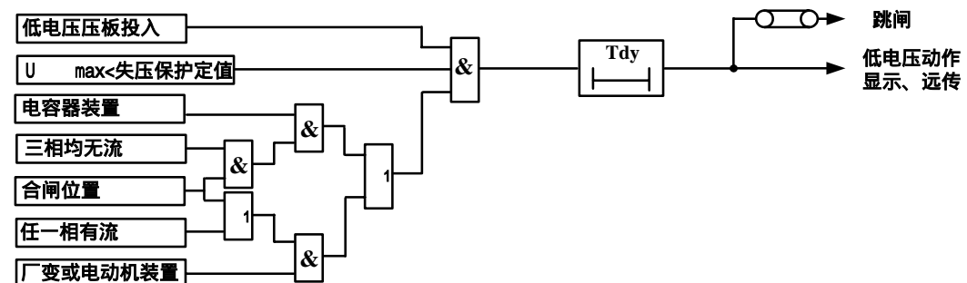
图 3-18 低电压保护原理框图
