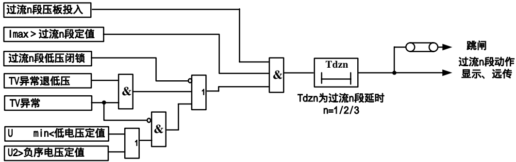
图 3-3 复压闭锁过流保护原理框图
