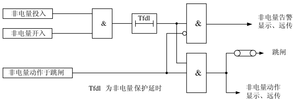
图 3-5 非电量保护原理框图
