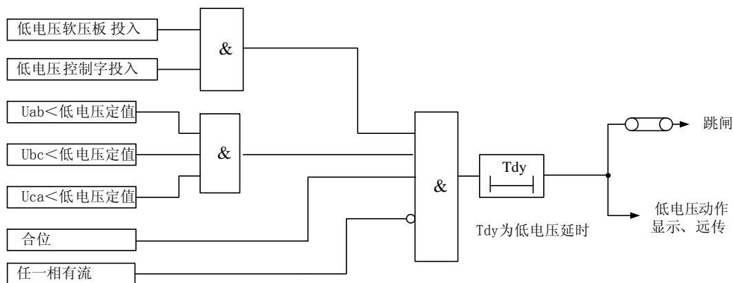
图 3-3 低电压保护原理框图
