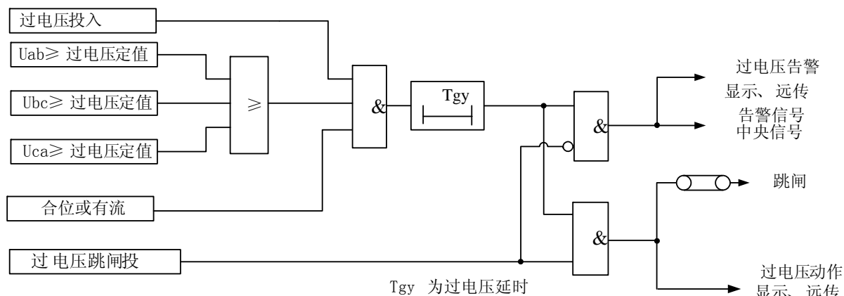
图 3-2 过电压保护原理框图
