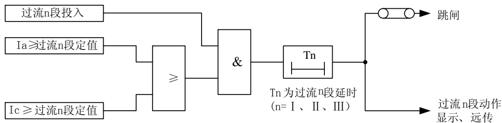
图 3-1 过流保护原理框图
