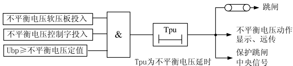
图 3-4 不平衡电压保护原理框图
